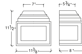
Corbel Plinth
