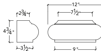
P-12B Plinth
